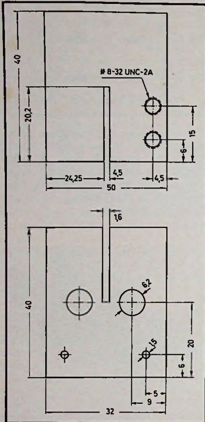
Bild 6. Abschirmbleche
