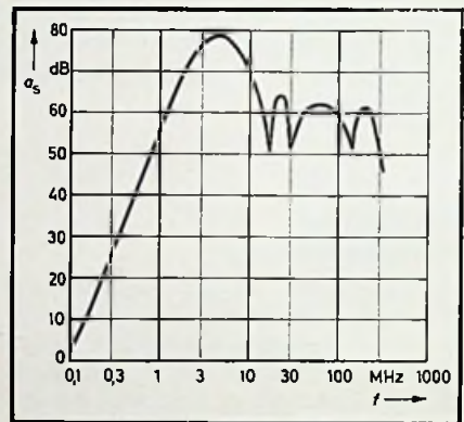
Bild 9. Dämpfungsverlauf des Netzfilters
