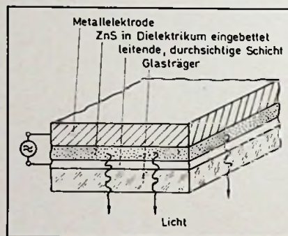
Bild 2. Schematischer Aufbau einer Elektrolumineszenzelle für Wechselspannung („Leuchtkondensator“)
