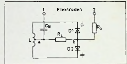
Bild 5. Schaltung eines miniaturisierten, passiven Senders für die Abnahme von Muskelpotentialen (nach Reilly 1968)
