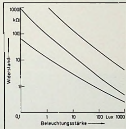
Bild 4. Typische Betriebswiderstände von CdS- und CdSe-Photoleitern
