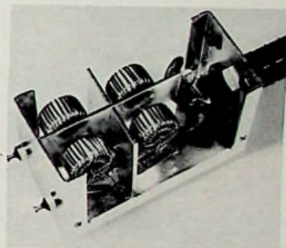
Bild 5. Netzfilter im geöffneten Zustand
