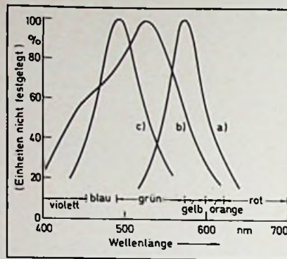
Bild 1. Emissionsspektrum einer mit Gleichstrom (a) und mit Wechselstrom (b) betriebenen ZnS-Elektrolumineszenzelle sowie einer LED aus ZnS_{1-x}Se_x (c)
