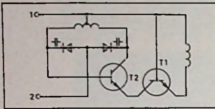
Bild 4. Schaltung eines implantierbaren Senders für die Abnahme von Muskelpotentialen. (1, 2 sind im Muskel liegende Elektroden) (nach Herberts, Kafors et al 1968)
